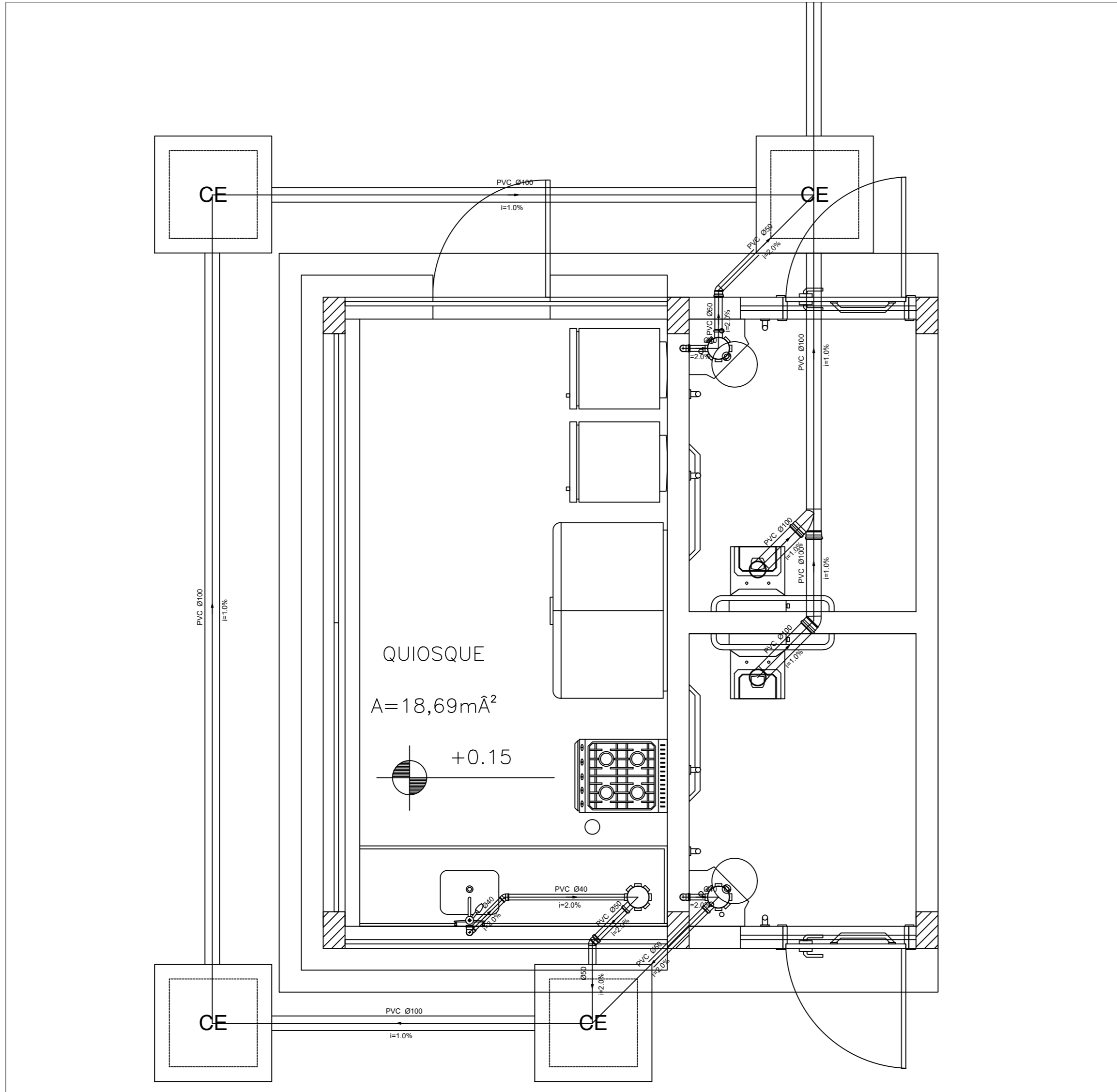
DETALHE 01 Campos, Maxaranguape/RN 1/20
